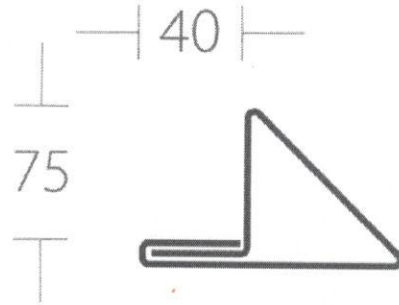
SNEGOBRAN
