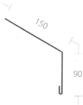
OKAPNICA
