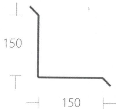
OPŠIVKA ZIDA
