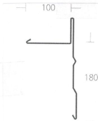
OKAPNICA
